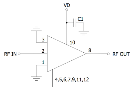
应用电路图
