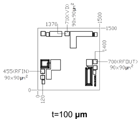
裸芯片外形尺寸( \mu\text{m} )
