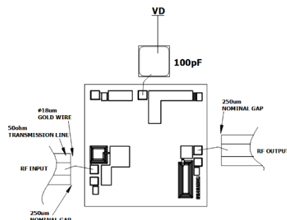
裸芯片推荐装配图
