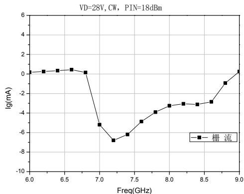
栅电流曲线
