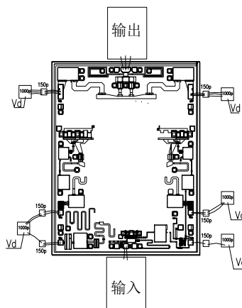
芯片装配示意图
