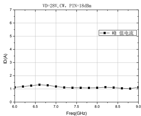
漏电流曲线
